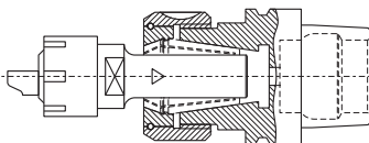
Optimale inspanlengte
